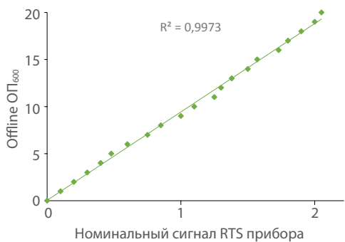
Рис. 7. Квадратичный коэффициент линейной корреляции (R 2 ) рассчитанных значений оптической плотности между данными полученными на RTS и на спектрофотометре (ОП 600 ). Калибровочная кривая получена для E.coli BL 21.
