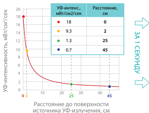
Рис. 1.1. Падение интенсивности УФ в зависимости от расстояния до источника УФ
