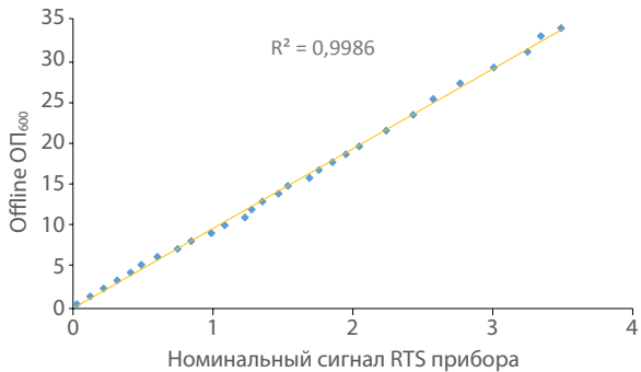
Рис. 8. Квадратичный коэффициент линейной корреляции (R 2 ) рассчитанных значений оптической плотности между данными полученными на RTS и на спектрофотометре (ОП 600 ). Калибровочная кривая получена для P.pastoris .
