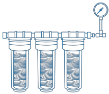
Externer Vorfiltersatz (Polyphosphat / Kohle / 1 µm) mit Manometer BS-070104-LK
